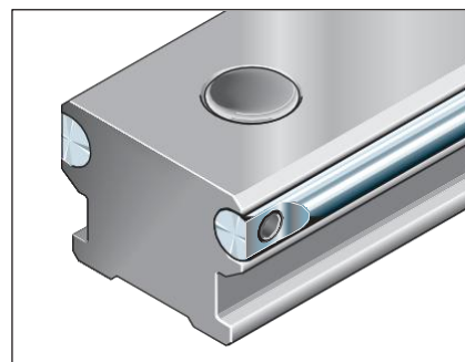
Rail de guidage standard Voies de guidage constituées d'arbres de précision en acier résistant à la corrosion
