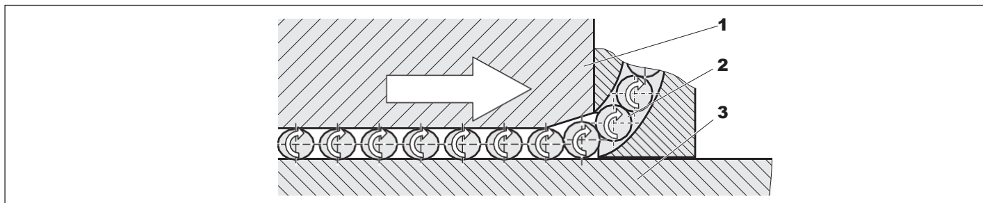
1 Guide à rouleaux 2 Rouleaux 3 Rail de guidage à rouleaux
